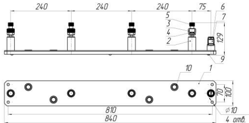
Рисунок 1- Коллектор К4-1000.
