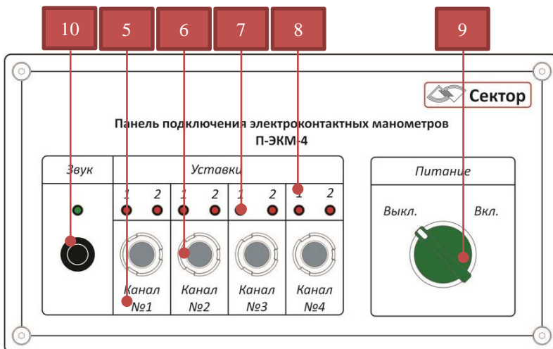
Рисунок 3. Передняя часть Панели П-ЭКМ-4
