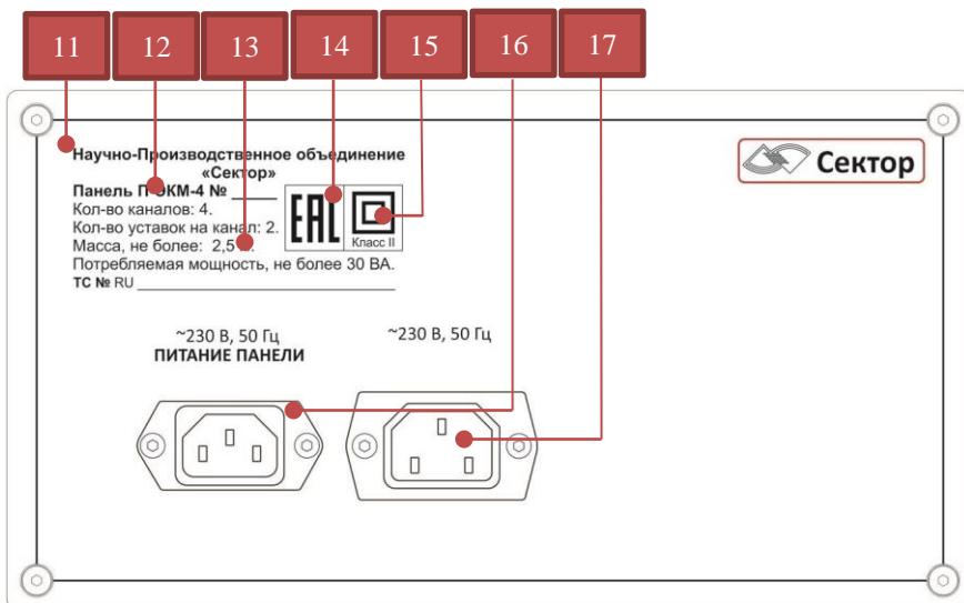
Рисунок 4. Задняя часть Панели П-ЭКМ-4
