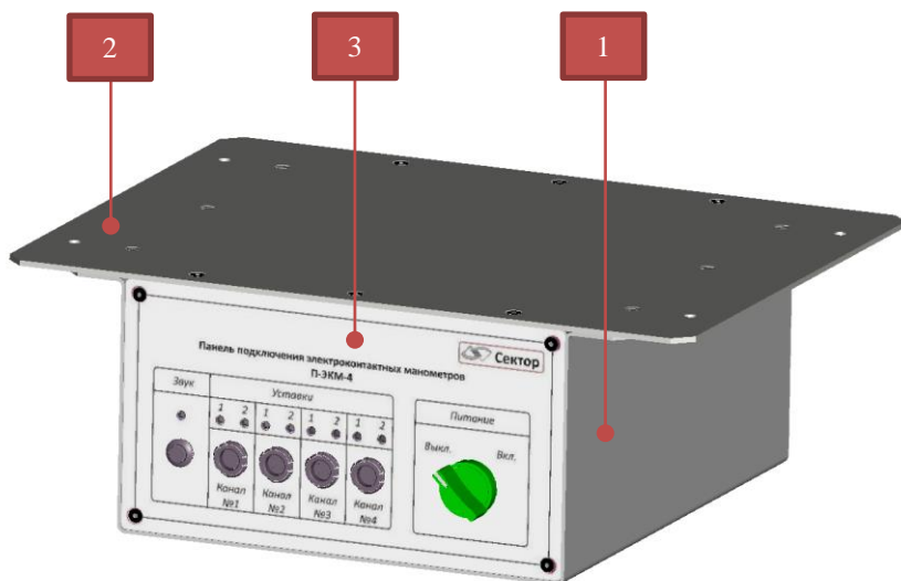
Рисунок 1. Панель П-ЭКМ-4 (вид спереди)
